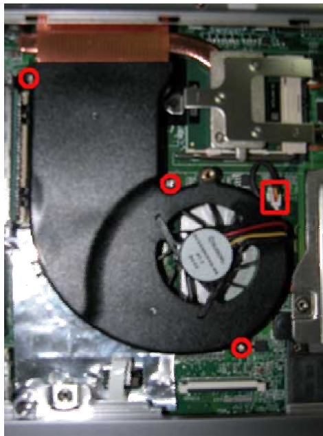
Fig. 21 CPU Fan
